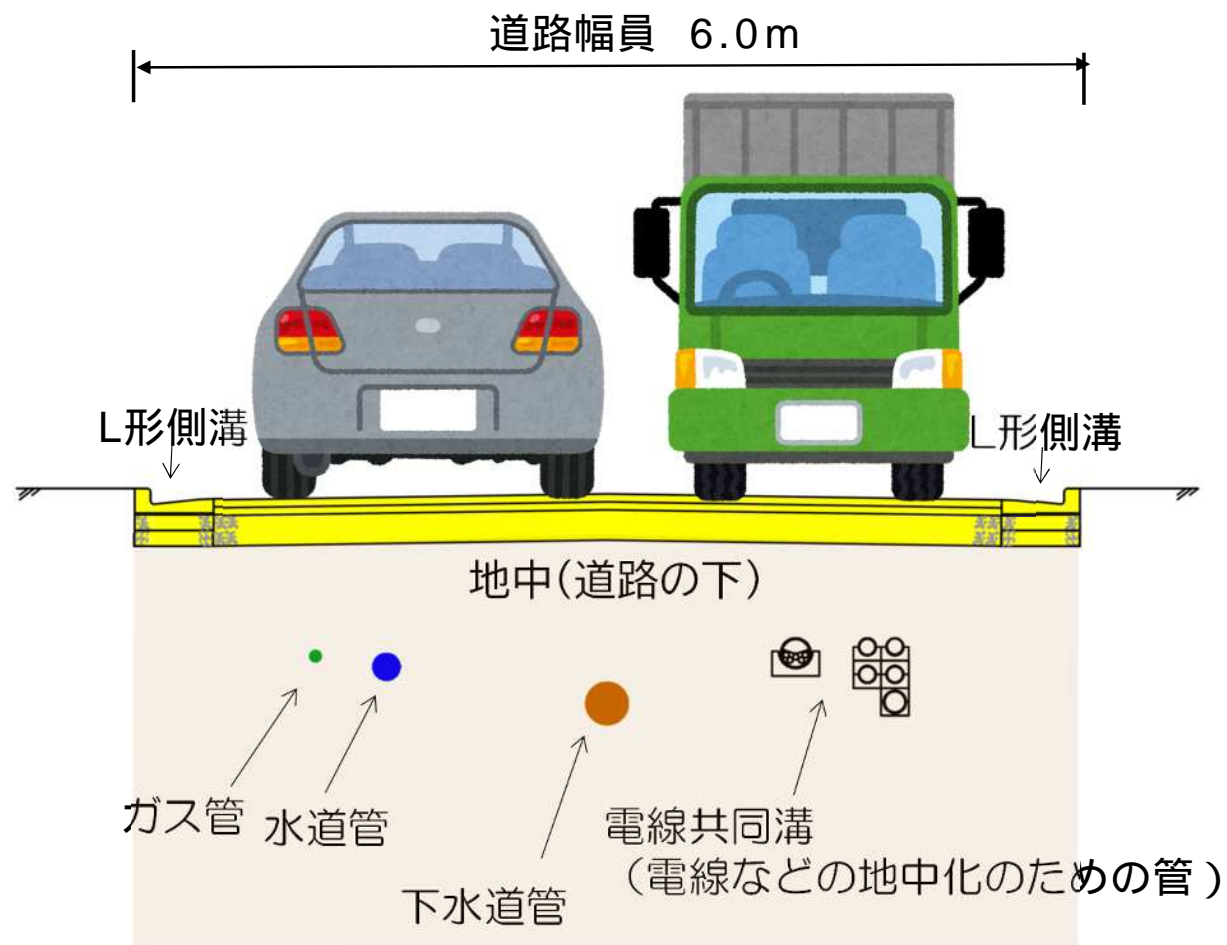
【断面図(A - A' 断面)】
