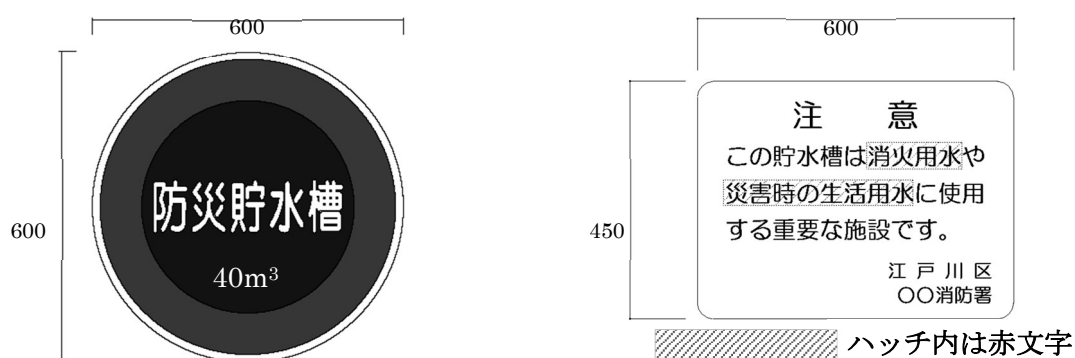
図3 防災貯水槽標識例
