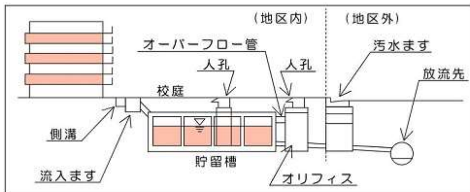
地下貯留施設の概念図
