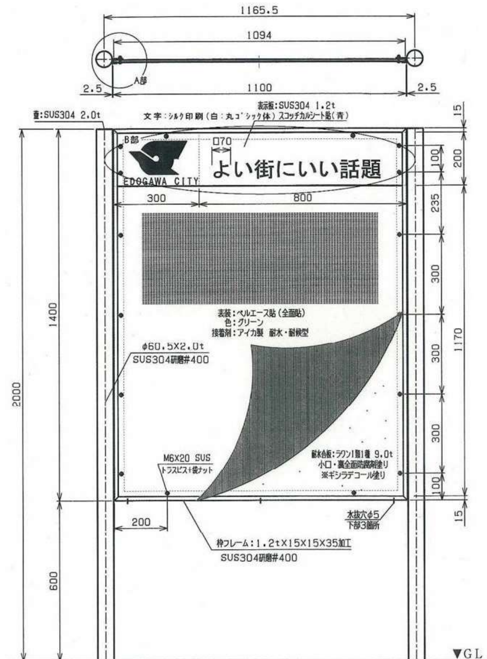
意匠図（前面・上面）
