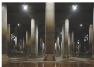
首都圏外郭放水路 調圧水槽（埼玉県春日部市）
