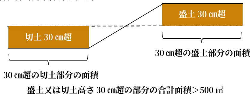
図 1-19 盛土又は切土する土地の面積が 500m 2 超で、盛土又は切土をする前後の地盤面の標高の差が 30cm 超となる場合のイメージ
