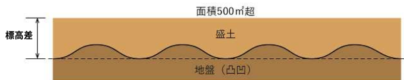
図 1-20 標高差の考え方
