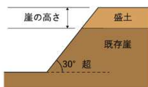
図 1-10 崖の高さ（盛土）
