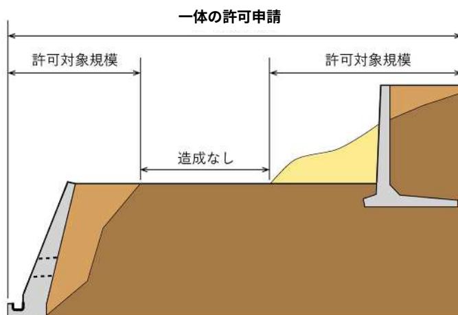
図 1-23 造成がない土地を間に挟む場合の許可対象行為②
