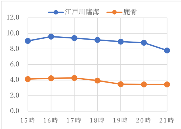
江戸川臨海(アメダス)と鹿骨観測点(東京都)の昨年7/25~8/3の15~21時風速の平均
