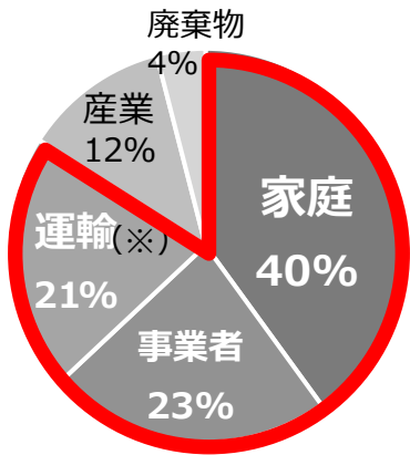
部門別CO2排出量(2018年度)
