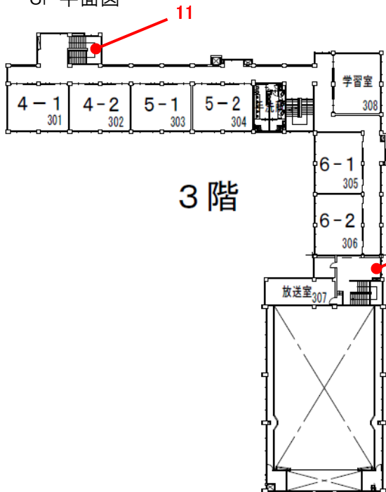
3F 平面図
