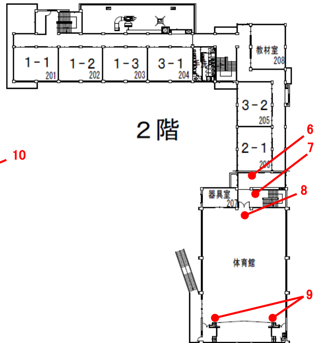
2F 平面図
